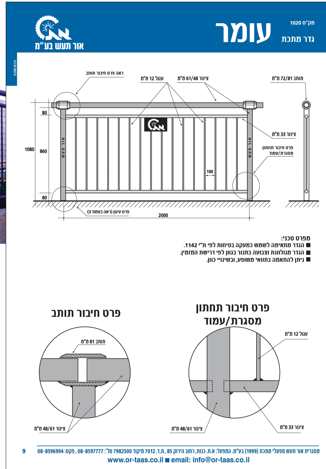
מעקה בטיחות קנ"מ 1:20
