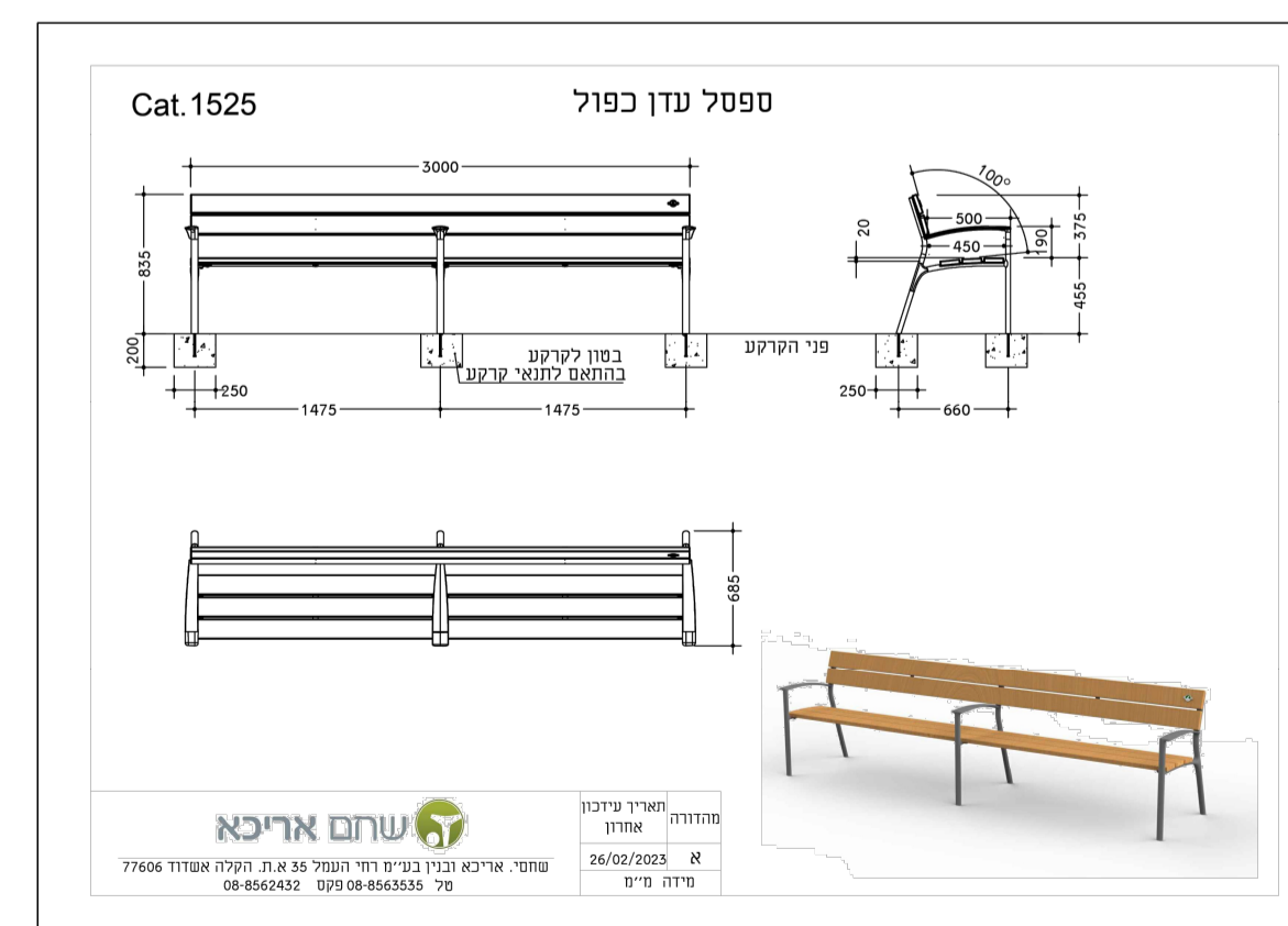
ספסל זוגי קנ"מ 1:20
