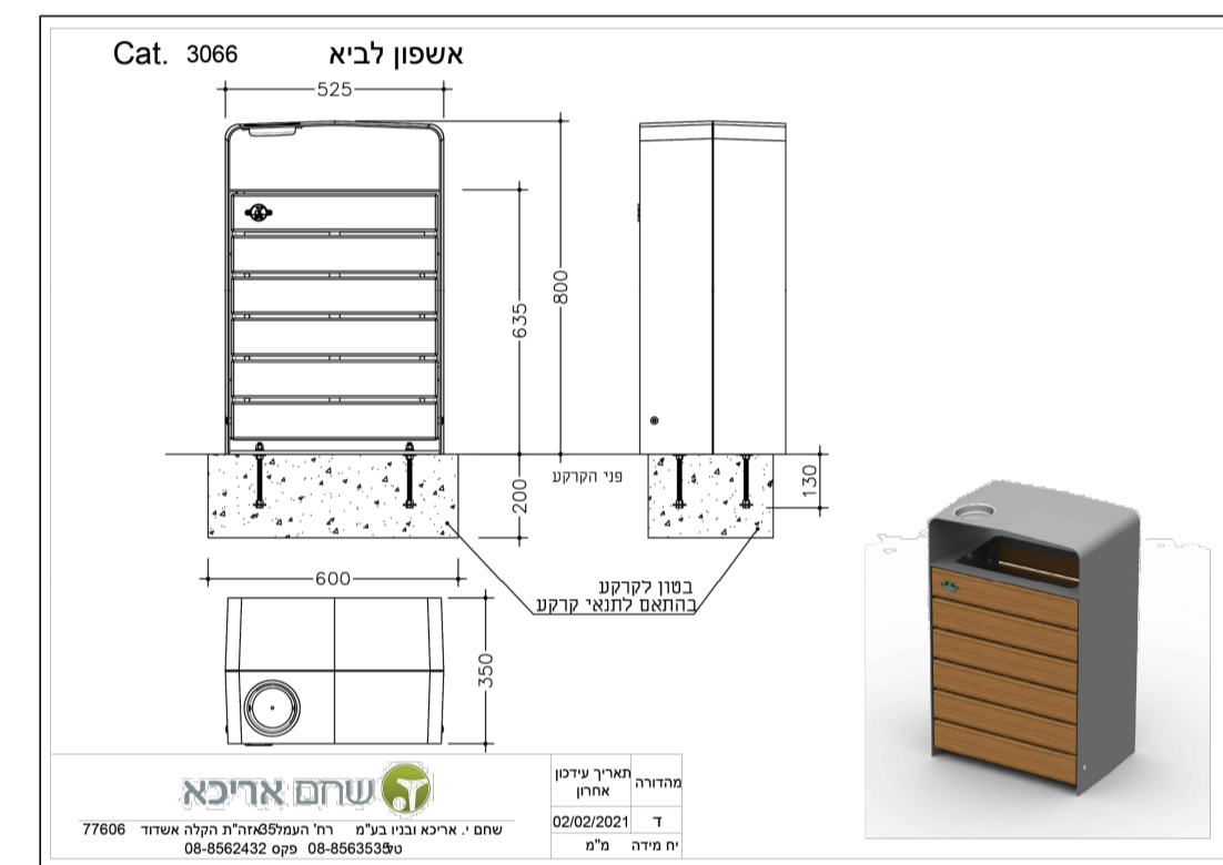
פח אשפה קנ"מ 1:20
