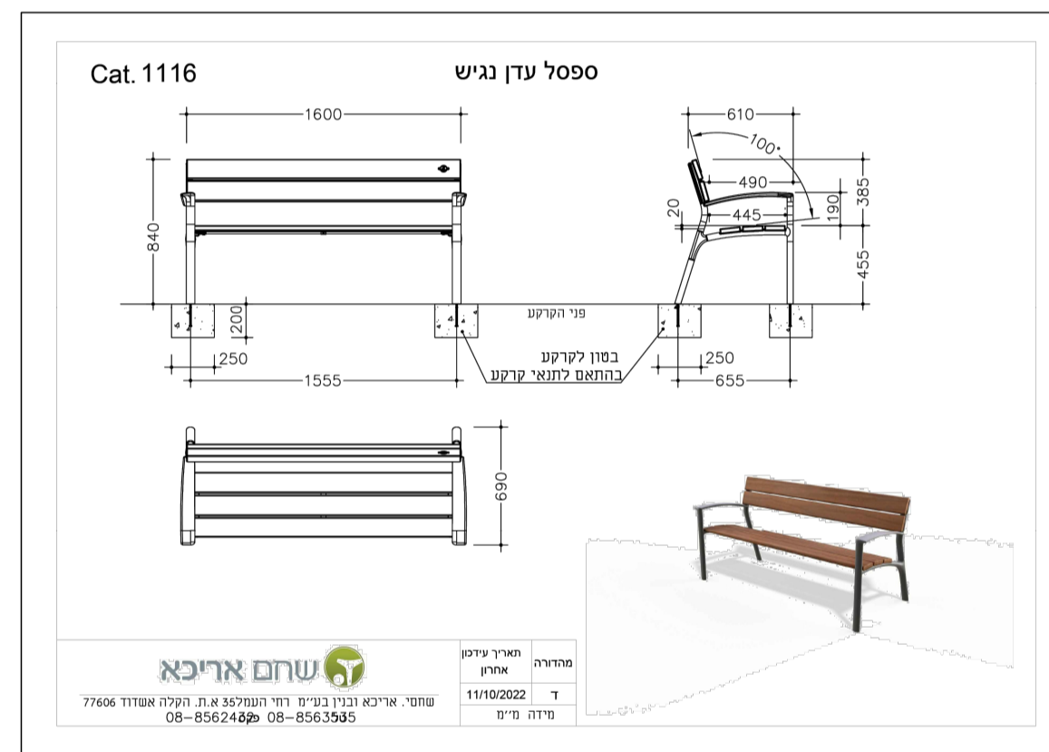
ספסל יחיד קנ"מ 1:20
