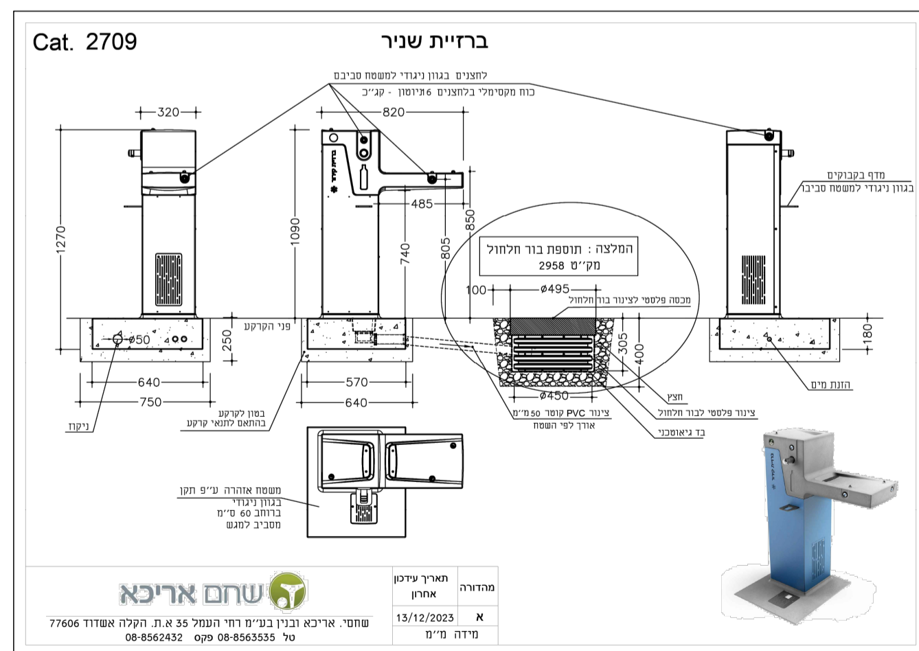
ברזייה קנ"מ 1:20
