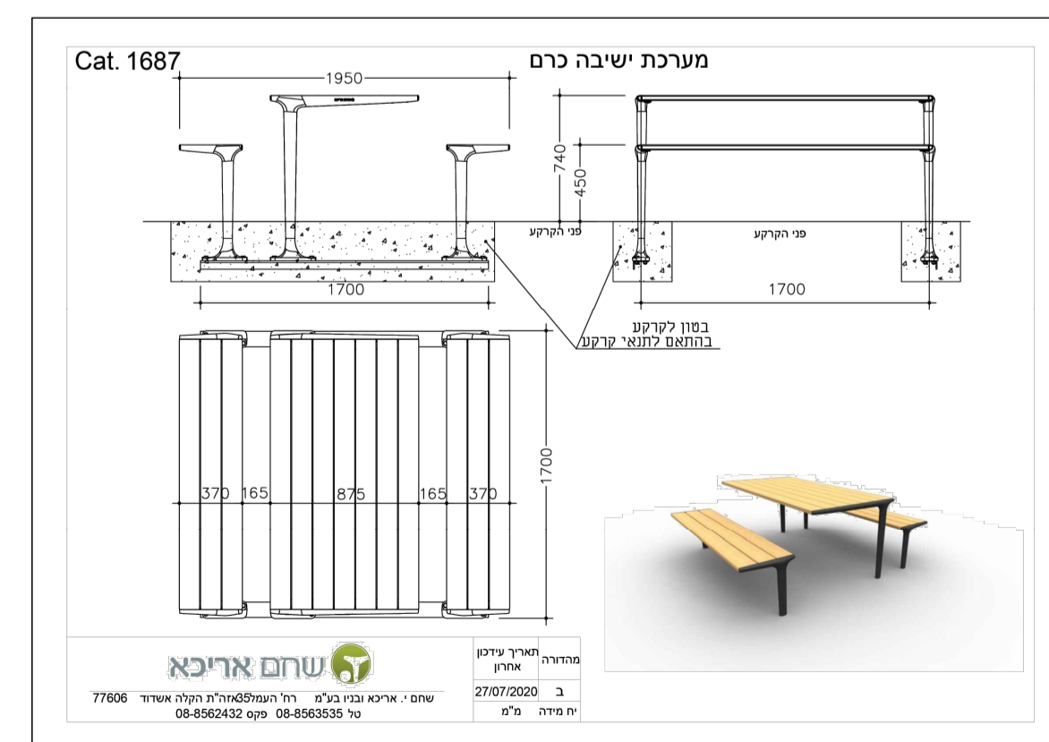
מערכת ישיבה נגישה קנ"מ 1:20
